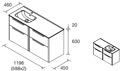
4 CAJONES CON LAVABO DESPLAZADO
