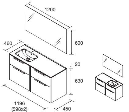
4 CAJONES CON LAVABO DESPLAZADO
